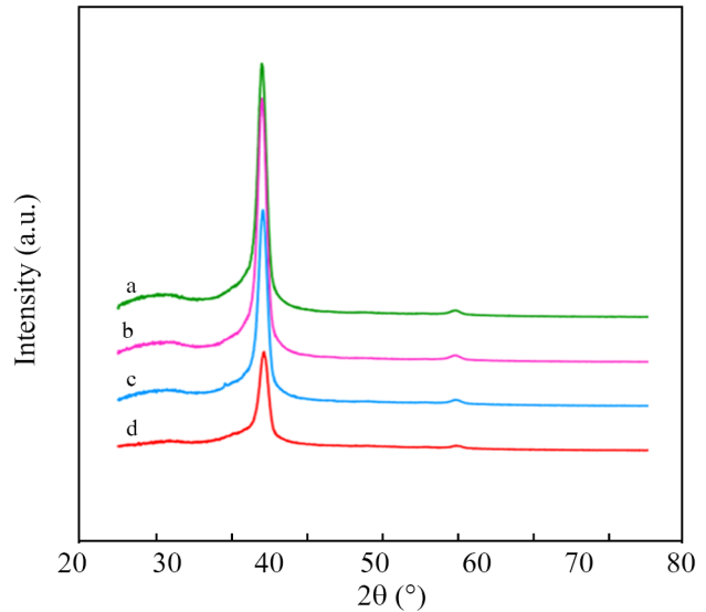
شکل ۵- الگوهای XRD غشاها: (a) Pebax خالص و Pebax-گلیسرول (b) ۵٪ وزنی، (c) ۱۵٪ وزنی و (d) ۲۵٪ وزنی.
