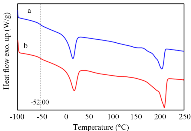
شکل ۶- دمانگاشت‌های DSC غشاها: (a) Pebax خالص و (b) Pebax-گلیسرول ۱۵٪ وزنی.
