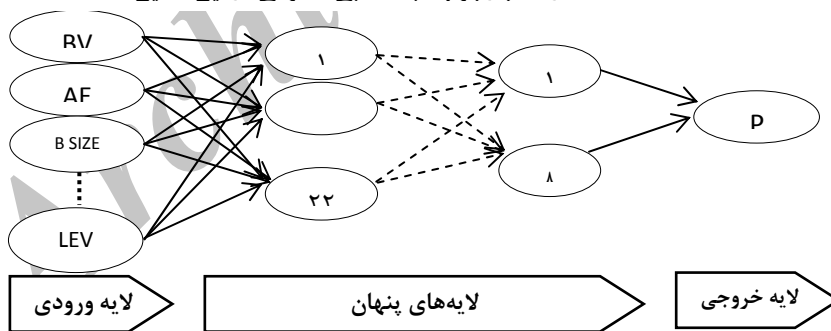
نگاره ۲: چارچوب شبکه عصبی مصنوعی در این تحقیق
