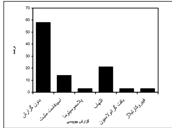
نمودار شماره ۳- درصد فراوانی نتایج بیوپسی در بیماران مبتلا به اسپوندیلیت و اسپوندیلودیسکیتیس بستری در بیمارستان‌های فیروزگر و حضرت رسول اکرم(ص) در سالهای ۸۲-۱۳۷۷
