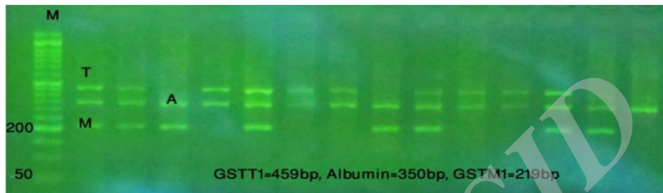
شکل ۱- محصول PCR ژن‌های GSTT1 و GSTM1 و Albumin بر روی ژل آگاروز چاهک M مارکر ۵۰ bp را نشان می‌دهد چاهک‌های ۱ تا ۱۴ ژن‌های تکثیر یافته را مشخص می‌کند. (M) ژن گلوکوتانیون S ترانسفراز، (T) ژن گلوکوتانیون S ترانسفراز، (A) آلبومین
