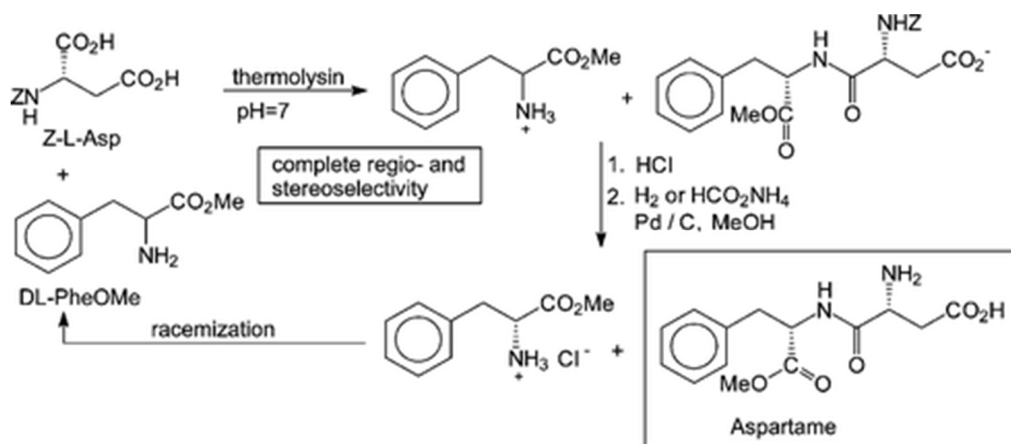
شکل ۳- روش آنزیمی تولید آسپارتام (۱۰)
