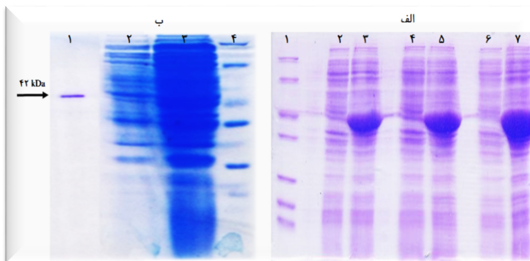
شکل ۳- الف) آنالیز بیان پروتئین کربوکسی پپتیداز G2 (۱: پروتئین مارکر - ۲: قبل القا زمان ۲ ساعت - ۳: بعد القا زمان ۳ ساعت - ۴: قبل القا زمان ۴ ساعت - ۵: بعد القا زمان ۴ ساعت - ۶: قبل القا زمان ۶ ساعت - ۷: بعد القا زمان ۶ ساعت). نمونه از ژل های الکتروفورز در زمانه های مختلف، دمای ۲۵ درجه سانتی گراد و غلظت ۰/۵ میلی مولار IPTG شکل ب) نمونه ۱: پروتئین تخلیص شده توسط ستون نیکل سفارز
