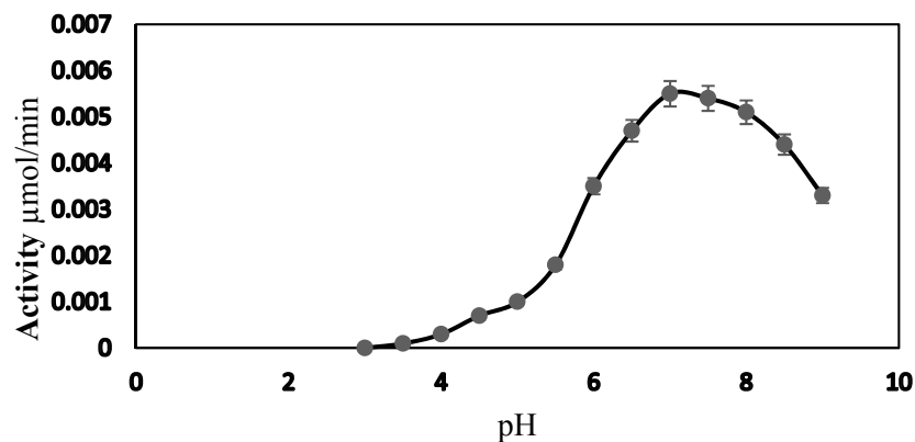
شکل ۴- تعیین pH بهینه- دمای بهینه الف) نمودار فعالیت- pH برای سوبسترای متوتروکسات در دمای محیط. و در مخلوط بافری حاوی تریس، سدیم فسفات، اسید سیتریک و گلايسين ۵۰ mM- در دامنه ۳-۹ pH مورد سنجش قرار گرفت. ب) نمودار فعالیت- دما برای سوبسترای - متوتروکسات در مخلوط بافری حاوی پتاسيم فسفات ۵۰mM
