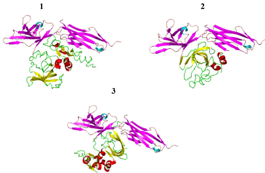
شکل ۲- مجموعه گیرنده و لیگاند نمایش داده شده توسط Discovery studio visualizer محصول آنالیز نتایج داکینگ مولکولی. ۱) HLMetInhibit1 بعنوان لیگاند و گیرنده ۲ فاکتور رشد اندوتلیال عروقی انسان بعنوان گیرنده (مولکول بنفش). ۲) HLMetInhibit2 بعنوان لیگاند و گیرنده ۳ فاکتور رشد اندوتلیال عروقی انسان بعنوان گیرنده (مولکول بنفش). ۳) Human TIMP-1 بعنوان لیگاند و گیرنده ۴ فاکتور رشد اندوتلیال عروقی انسان بعنوان گیرنده (مولکول بنفش)
