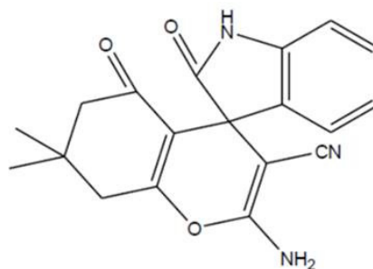
شکل ۱- ۲- آمینو-۷-دی متیل-۵-دی اکسو-۵-هکسوفو-۸-تراهیدرو اسپایرو {۳-ایندولین-۳-کربونیتیل
