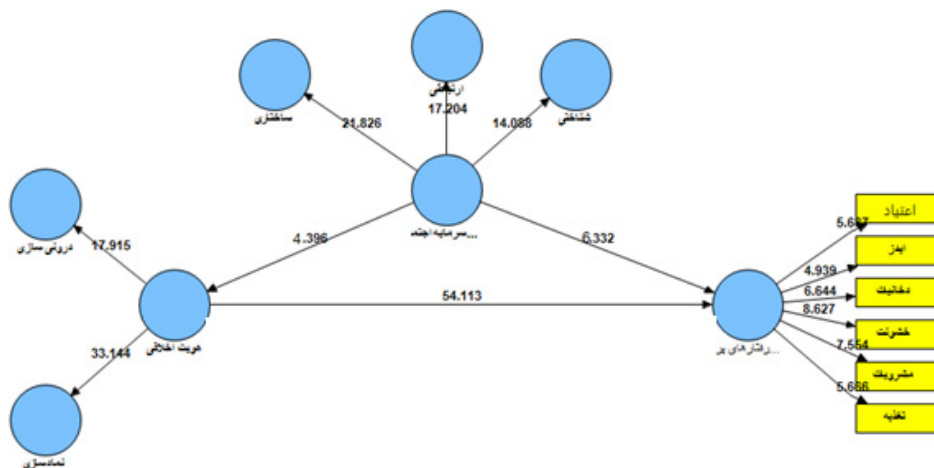
شکل ۳- ضرایب معنی داری t (مقادیر t-values)
