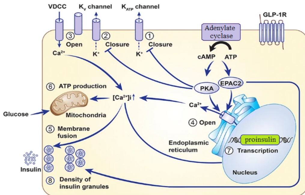
شکل ۱- مکانیسم‌های مولکولی زمینه‌ساز اثرات انسولینوتروپیک GLP-1 (۶۲) مکانیسم‌های مولکولی در بندهای ۱ تا ۸ در توضیحات فوق مطرح شده است.
