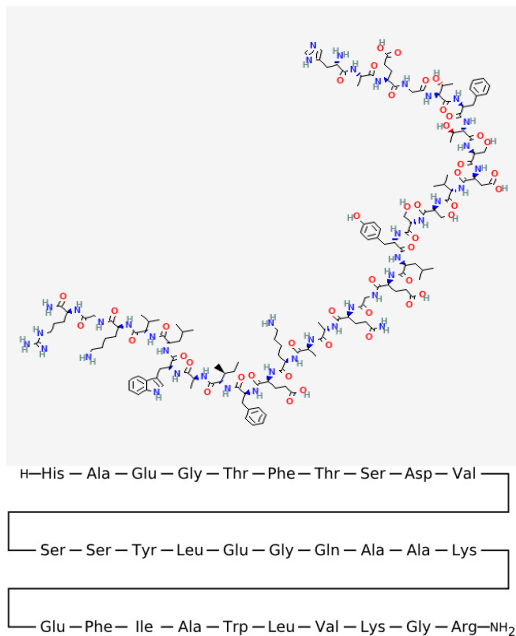
شکل ۲- ساختار دومی و توالی GLP-1 برگرفته از PubChem
