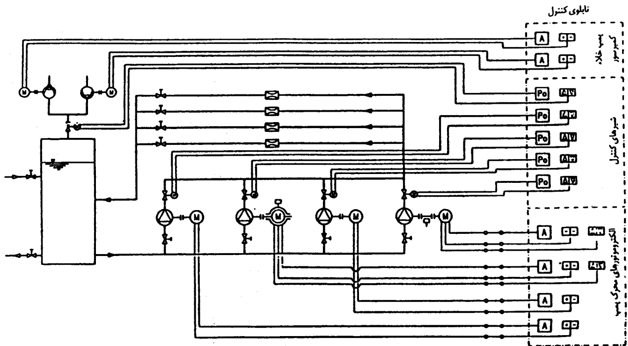
شکل ۷: مدار شماتیک آزمایش کایتاسیون پمپ سانتریفوژ.
