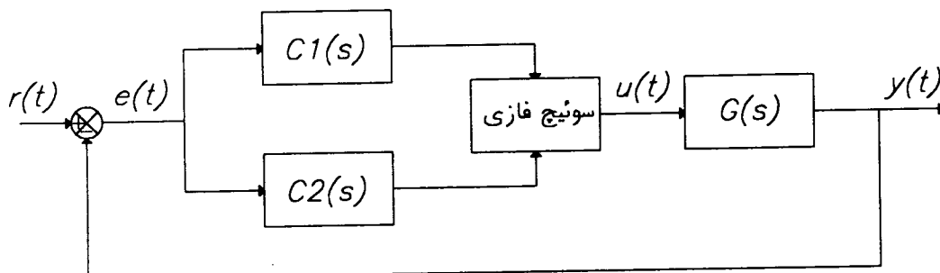
شکل ۴: نمایش کنترل کننده خطی - فازی به صورت دو کنترل کننده خطی و یک سوییچ فازی.
