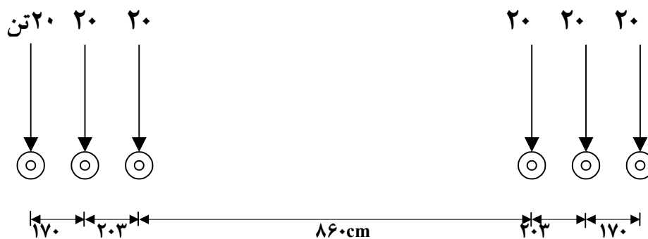
شکل ۱۰: شبیه سازی بار دیزل ۱۲۰ تنی ۶ محوره به صورت تنش بار متحرک.
