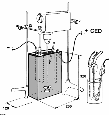
شکل ۲: نحوه نصب تجهیزات مورد نیاز آزمایش.
