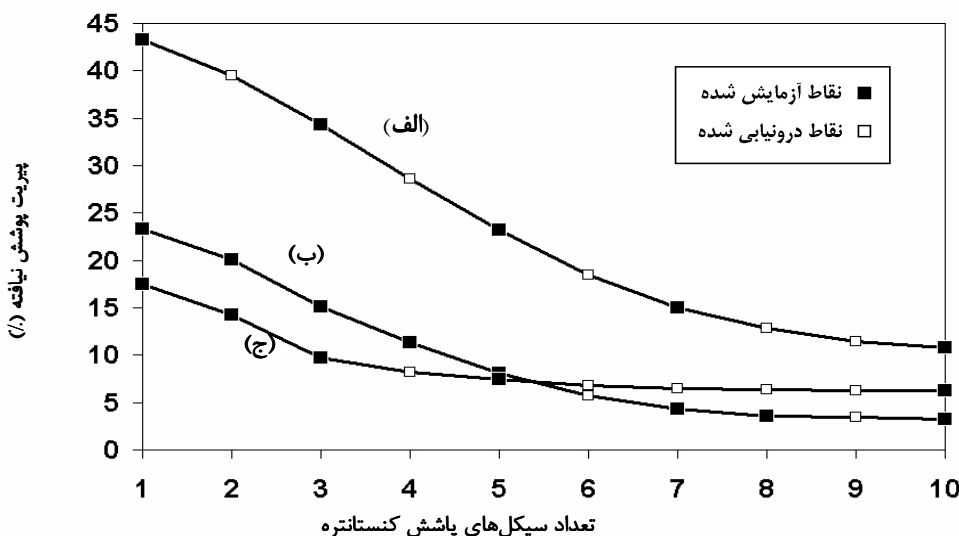
شکل ۱: تغییرات میزان کنسانتره پوشش نیافته نسبت به تعداد سیکل و درجه انباشستگی.
