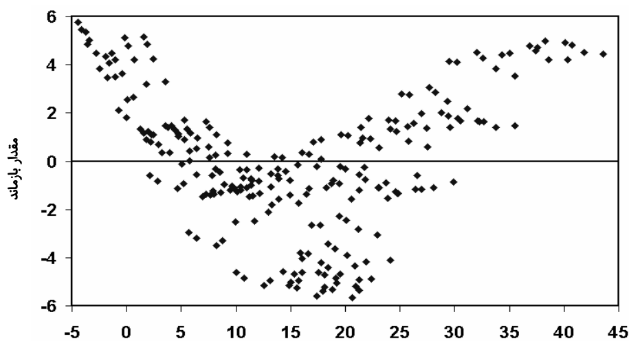
شکل ۴: نمودار مقادیر بازماند در مقابل مقادیر پراش داده شده. ANOVA
