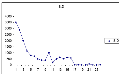
شکل ۱۰: تغییرات انحراف معیار ۲۴ نسل مربوط به مسأله ۱۰×۱۲ بدون در نظر گرفتن هزینه انتقالات درون سلولی .
