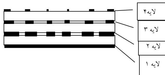
شکل ۱۲: شکل مقطع ساختار FZPA چهار لایه P = 4 .
