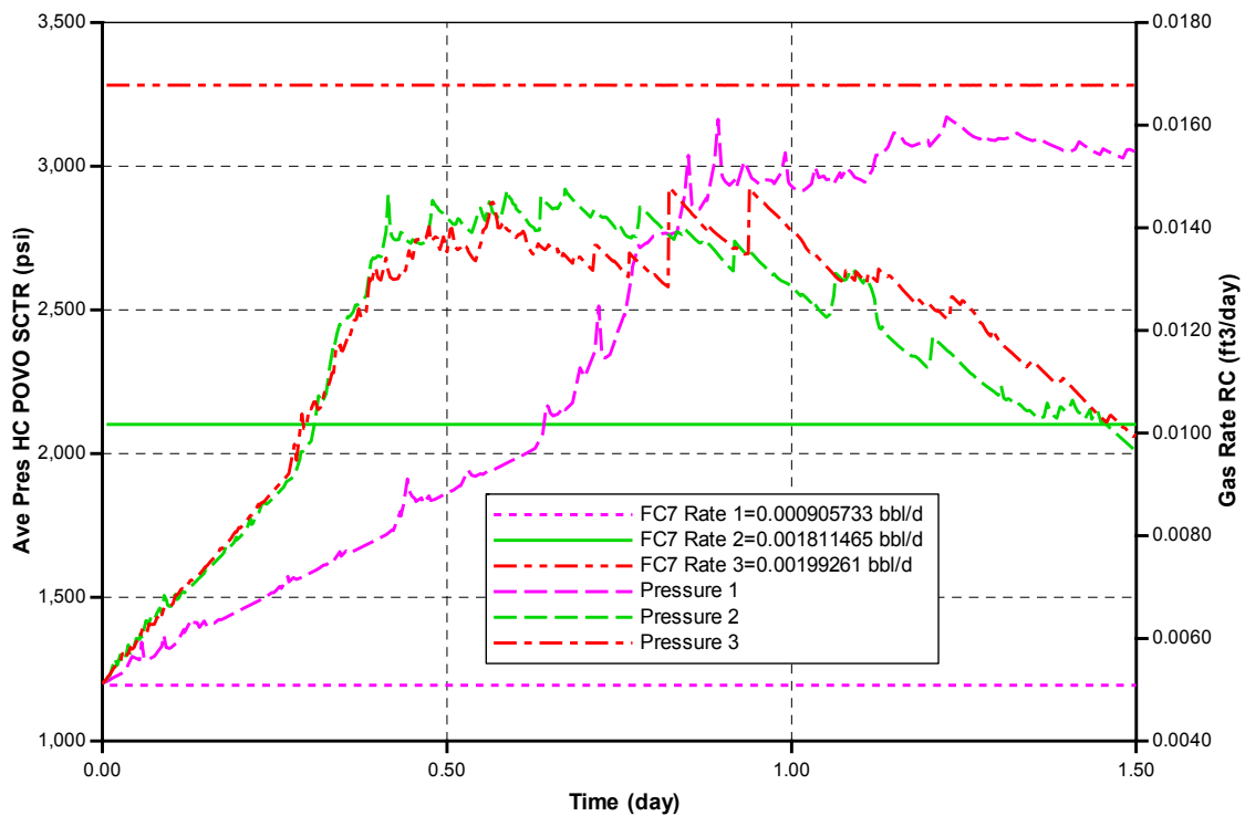
شکل ۱۴: مقایسه اثر تغییر دبی نرمال هیتان تزریقی بر افزایش فشار میانگین مخزن.
