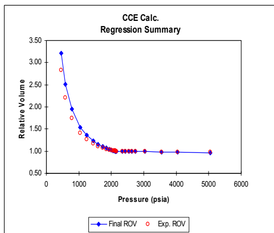
شکل ۱۱: نتایج تطابق داده های آزمایشگاهی حجم نسبی نفت و جوابهای معادله حالت برای آزمایش تبخیر با ترکیب ثابت.
