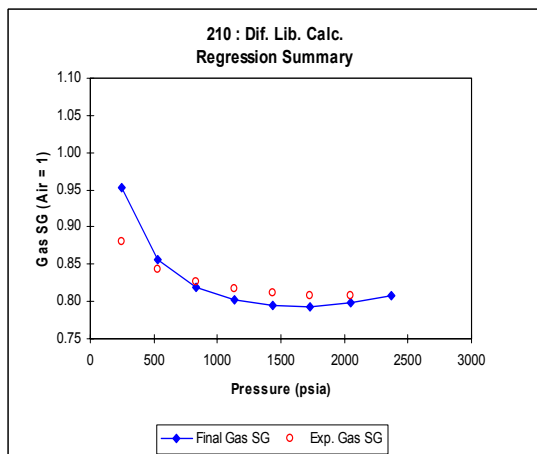
شکل ۶: نتایج تطابق داده های آزمایشگاهی وزن مخصوص گاز و جوابهای معادله حالت برای آزمایش تبخیر تفاضلی در 210^{\circ}\text{F} .
