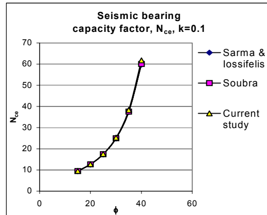
شکل ۴: مقایسه ضریب ظرفیت باربری N_{ce} برای K=0.1 .
