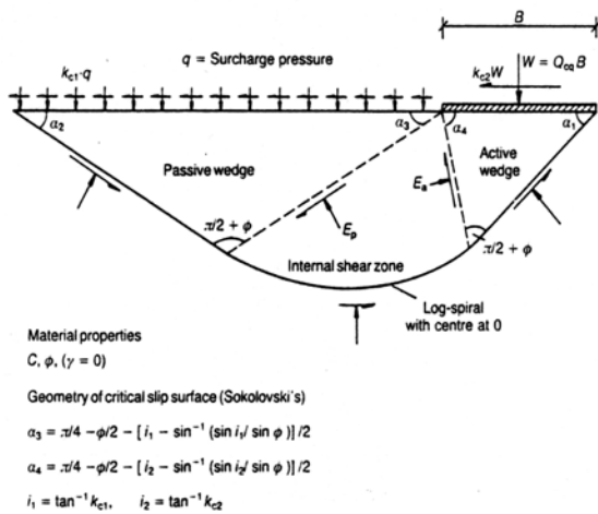
شکل ۲: جزئیات مکانیزم مورد استفاده توسط سارما و یوسفلیس (Sarma & Iossifelis 1998).
