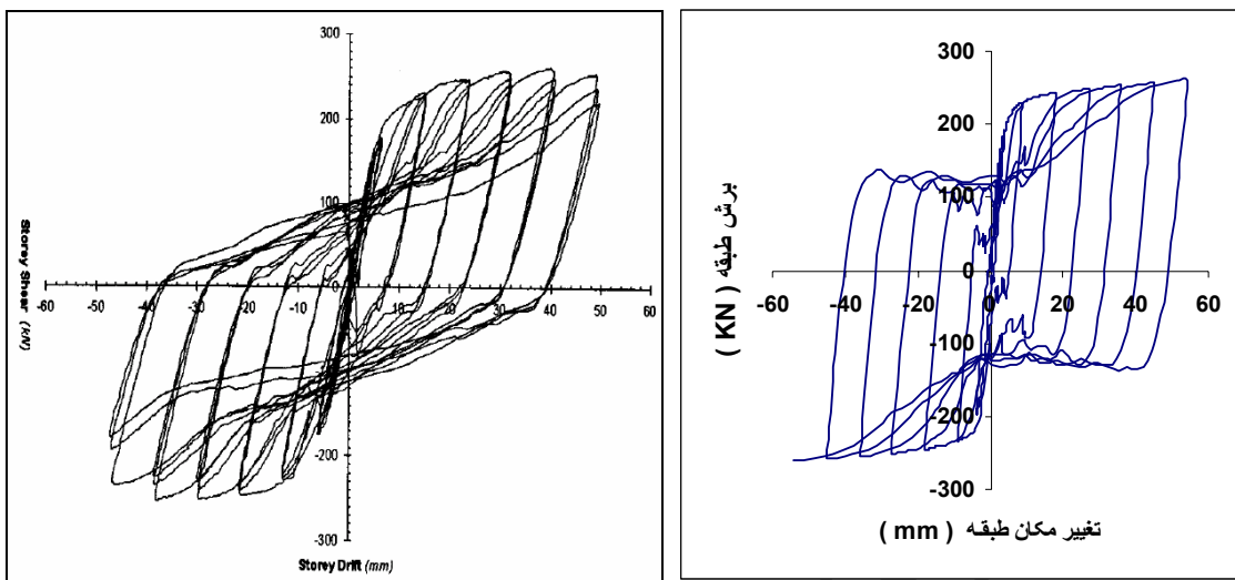
شکل ۶: منحنی هیستریزیس بدست آمده از تحلیل کامپیوتری (سمت راست) آزمایش [۴] (سمت چپ).
