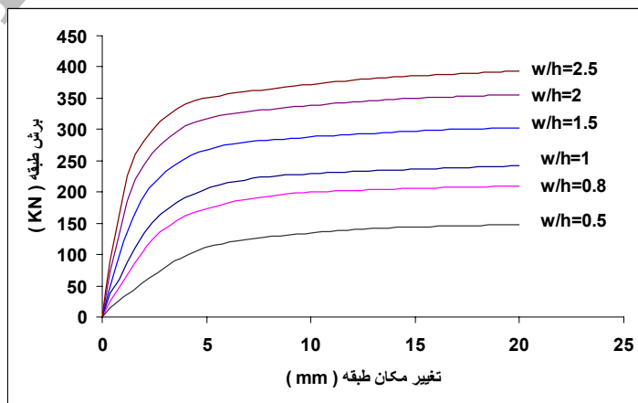
شکل ۱۴: تاثیر نسبت عرض دهانه به ارتفاع طبقه در مقاومت سیستم.
