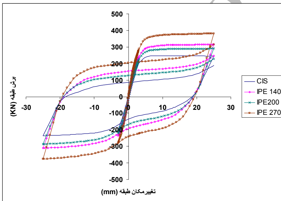
شکل ۱۱: تاثیر سختی ستون بر رفتار هیستریزیس.
