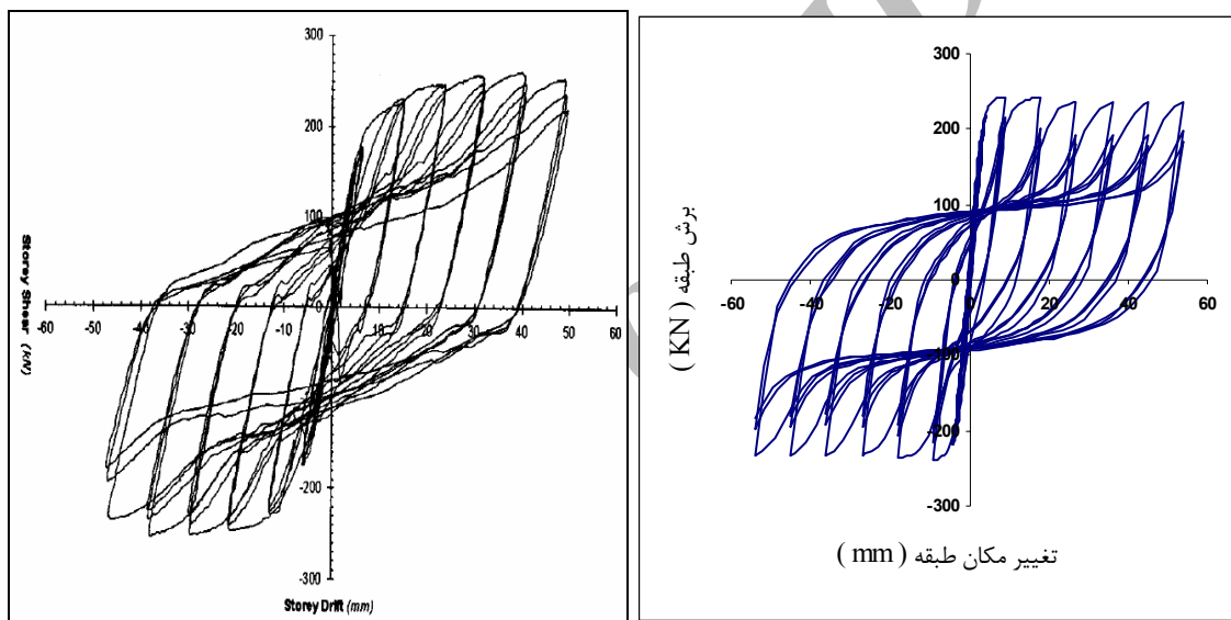
شکل ۸: منحنی هیستریزیس بدست آمده از تحلیل کامپیوتری (سمت راست) آزمایش [۴] (سمت چپ).
