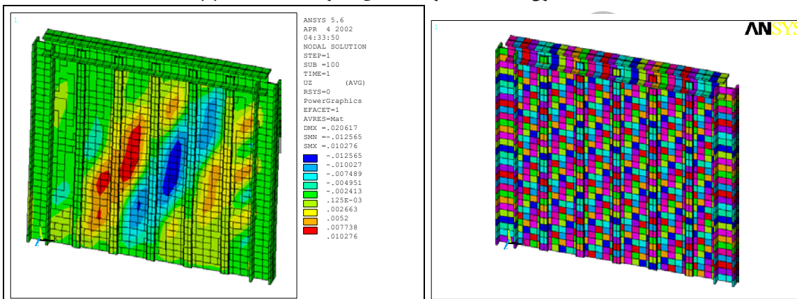
شکل ۱۶: مدل سخت کننده دار (راست) نمای تغییر شکل یافته مدل (چپ).
