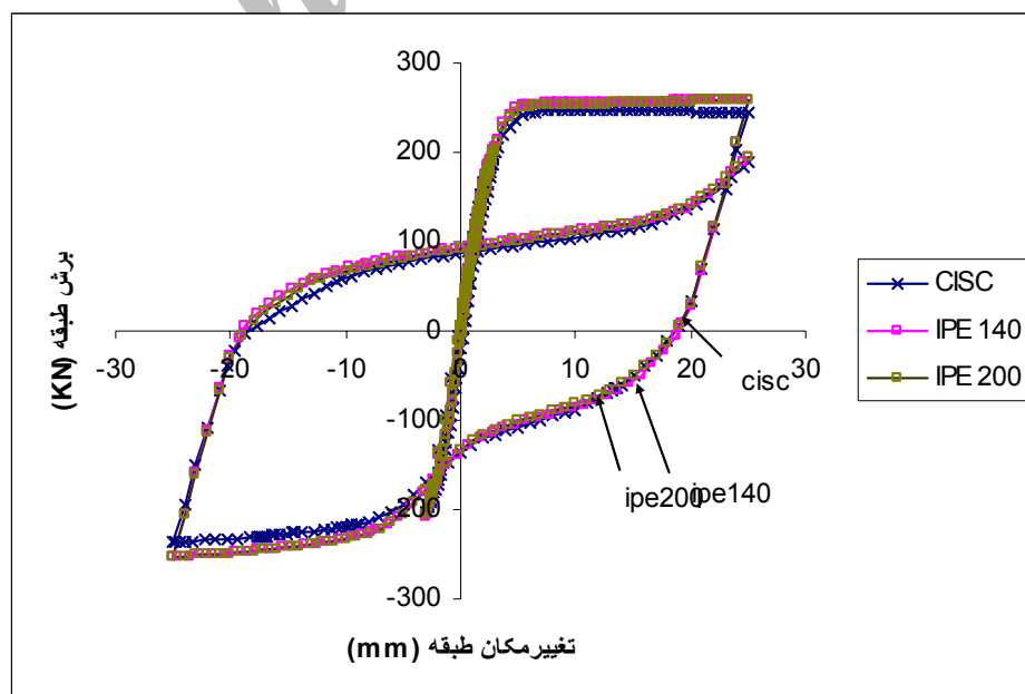
شکل ۱۲: تأثیر سختی تیر بر رفتار هیستریزیس.
