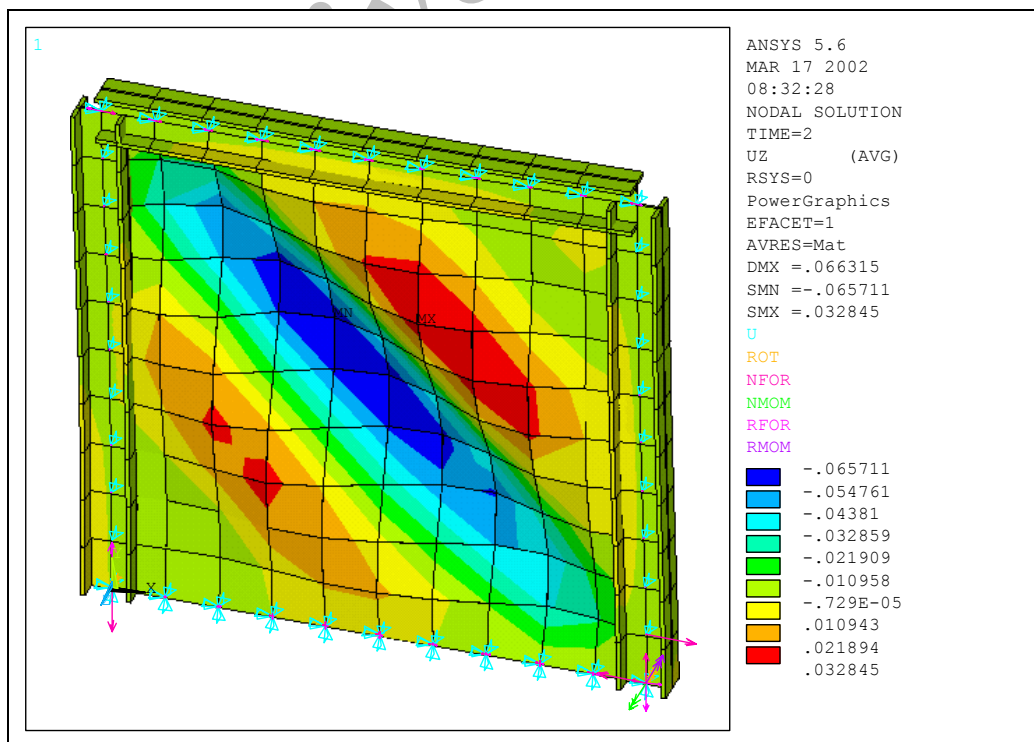
شکل ۵: مدل تغییر شکل یافته.
