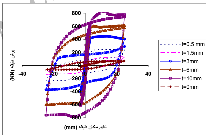
شکل ۹: تغییر رفتار هیستریزیس با افزایش ضخامت ورق.
