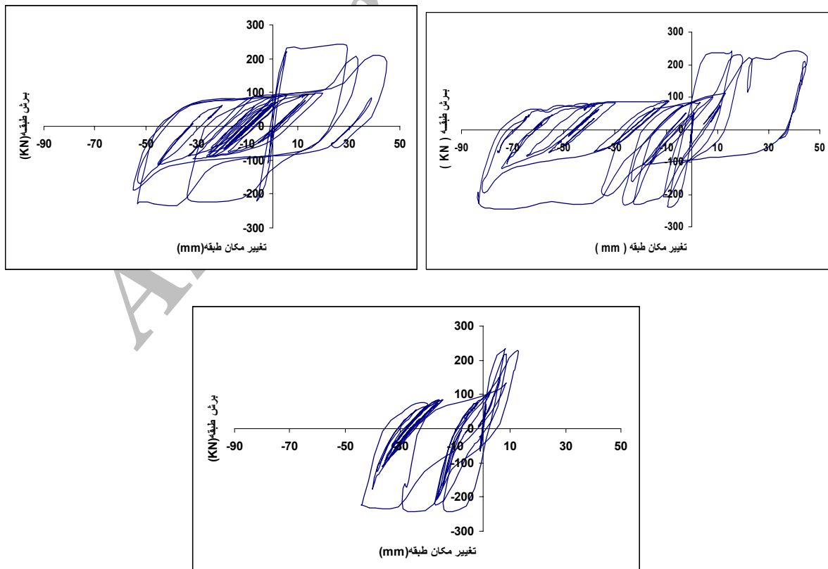
شکل ۱۸: منحنی هیستریزس زلزله های طبس (بالا) السنترو (وسط) منجیل (پایین).
