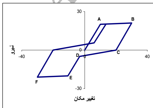
شکل ۲: منحنی هیستریزس دیوار برشی فولادی.
