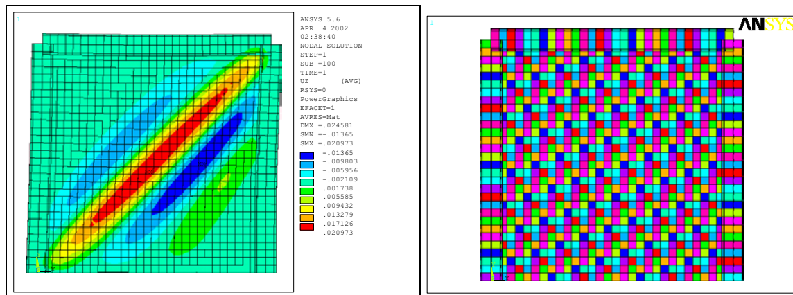
شکل ۱۵: مدل بدون سخت کننده (راست) نمای تغییر شکل یافته مدل (چپ).
