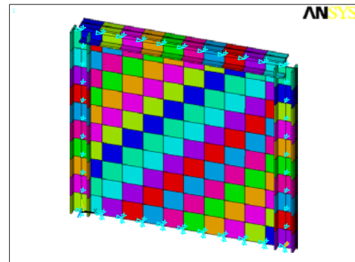
شکل ۴: نمونه مدلسازی شده در برنامه ANSYS.
