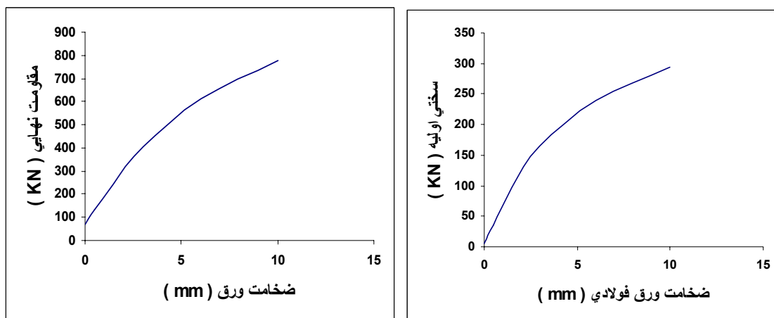
شکل ۱۰: تاثیر ضخامت ورق فولادی بر پارامترهای مقاومت.
