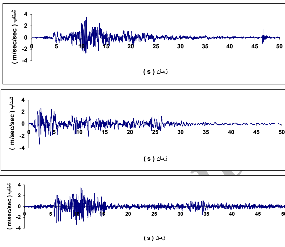
شکل ۱۷: شتاب نگاشت مقیاس شده زلزله های طبس (بالا) السنترو (وسط) منجیل (پایین).
