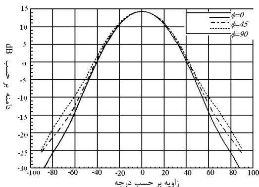
شکل ۱۴: بهره محاسبه شده توسط نرم افزار Ansoft HFSS برای شیپوری با ساختار نامنظم شیارها.
