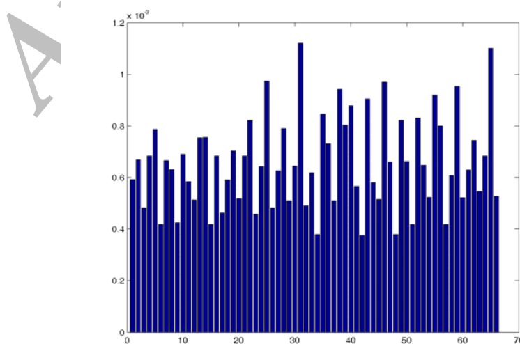
شکل ۴: انحراف معیار مختصات نقاط حاصل از سرشکنی (بر حسب متر).
