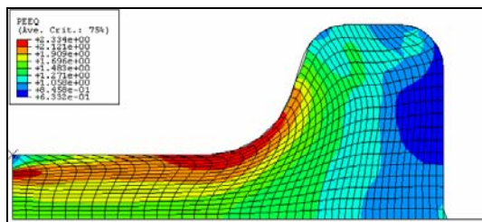
شکل ۸: کانتور توزیع کرنش پلاستیک معادل در پایان فرآیند آهنگری دو مرحله ای.
