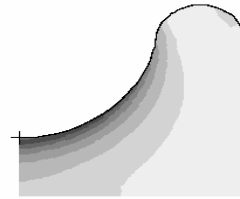
شکل ۹: کانتور توزیع کرنش پلاستیک معادل در پایان فرایند آهنگری دو مرحله ای [ مرجع ۱۲ ].
