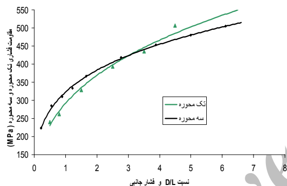
شکل ۱۵: بر هم نهی نمودارهای حاصل از آزمون های تک محوره و سه محوره برای ماسه سنگ گدوک.
