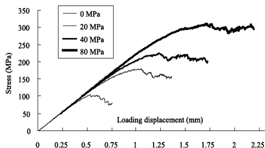
شکل ۳: تاثیر فشار جانبی بر مقاومت فشاری تک محوره [۳].
