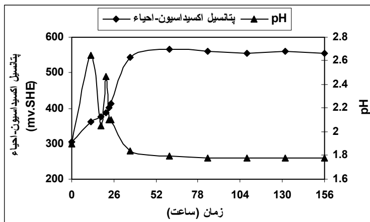
شکل ۷: تغییرات پتانسیل اکسیداسیون-احیاء و اسیدیته پالپ در راکتور همزن‌دار (محیط کشت = 9K، درصد میزان جامد پالپ = ۵ درصد، میزان تلقیح = ۱۰ درصد).
