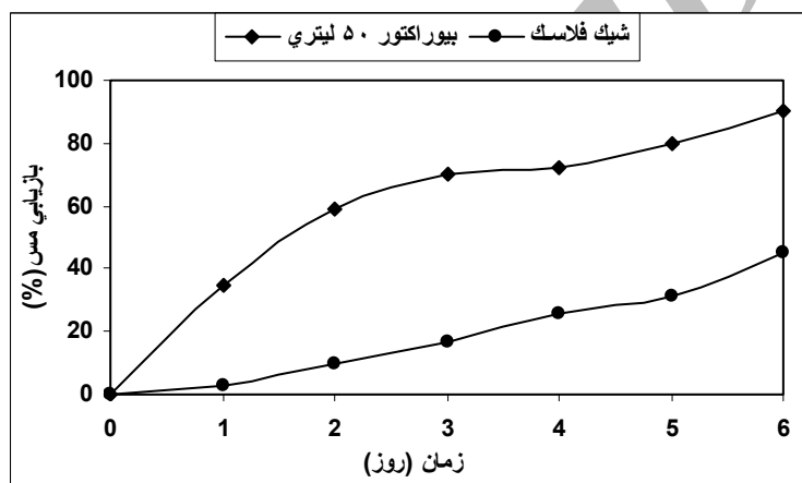
شکل ۸: تاثیر نوع راکتور بر بازیابی مس در فرایند انحلال زیستیغبار (محیط کشت = 9K، درصد میزان جامد پالپ = ۵ درصد، میزان تلقیح = ۱۰ درصد).
