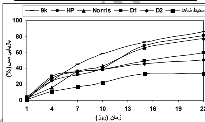
شکل ۱: تاثیر نوع محیط کشت بر میزان بازیابی مس (درصد میزان جامد پالپ = ۵ درصد، میزان تلقیح = ۱۰ درصد).
