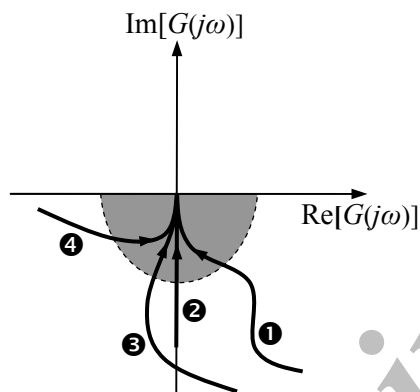
شکل ۱: دیاگرام نایکویست G(j\omega) با درجه نسبی یک فرکانس های به اندازه کافی بزرگ.
