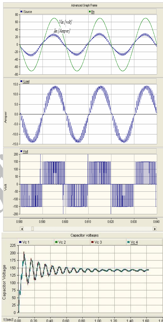
شکل ۱۲: ولتاژهای ورودی و خروجی به همراه جریانهای ورودی و خروجی مبدل و کنترل حلقه بسته ولتاژهای DC با میزان مرجع 141.41 \text{ V} با OC=25\% در فرکانس سویچینگ 2000 \text{ Hz} .
