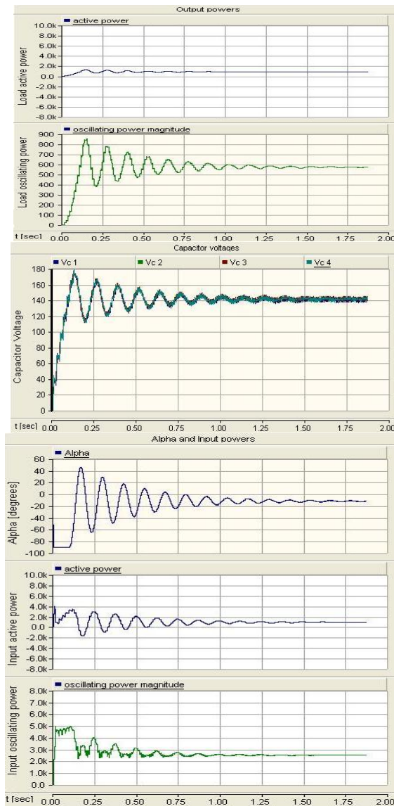
شکل ۱۱: کنترل حلقه بسته ولتاژهای DC با میزان مرجع V_{dc}^* = 141.41 V (a) ، تنظیم زاویه \alpha توسط کنترلر، توان متوسط اکتیو و اندازه توان نوسانی هارمونیک دوم ورودی، (b) توانهای اکتیو و نوسانی هارمونیک دوم بار، (c) وضعیت تعادل ولتاژهای DC چهار مدول با تغییرات ولتاژ زیر ۳ ولت.
