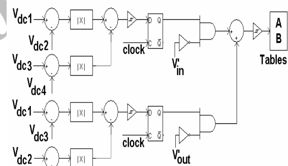
شکل ۶: نحوه اجرایی کردن انتخاب یکی از دو جدول (a-۳) یا (b-۳) با توجه به متعادل ساختن ولتاژ خازنها.
