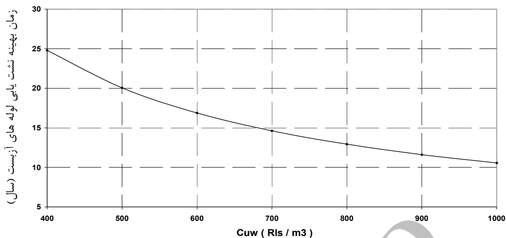
شکل ۶: آنالیز حساسیت زمان نشت یابی لوله های آریست نسبت به پارامتر C_{uw} .
