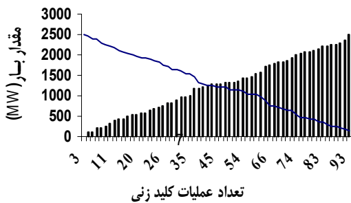
شکل ۱۰: منحنی اختصاص تولید به بارهای مصرفی جزیره ۲.
