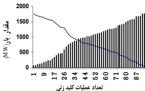
شکل ۹: منحنی اختصاص تولید به بارهای مصرفی جزیره ۱.
