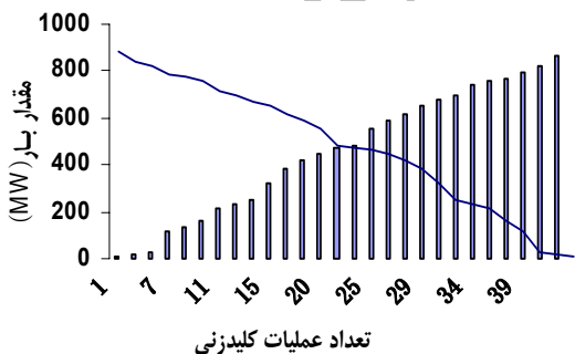
شکل ۲۰: منحنی اختصاص تولید به بارهای مصرفی جزیره ۱.
