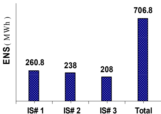
شکل ۱۸: مقادیر ENS جزیره‌های ۱، ۲، ۳ و ENS کل شبکه.
