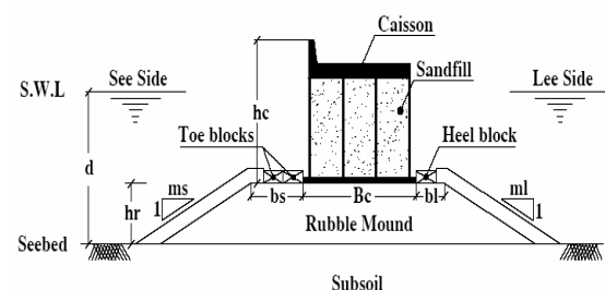
شکل ۱: مشخصات هندسی موج‌شکن مرکب.
