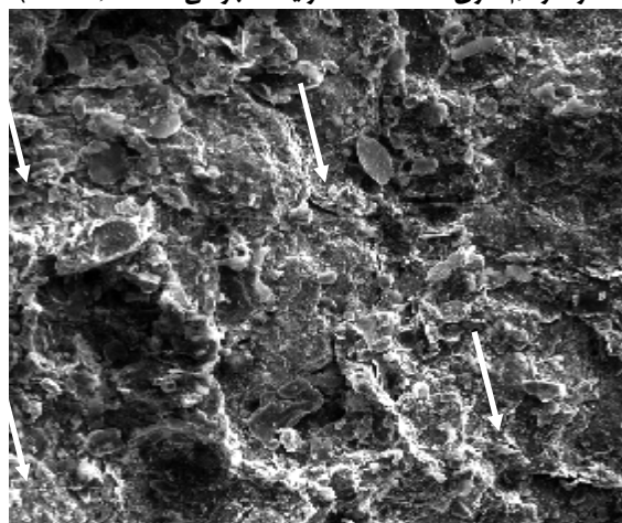
شکل ۶: تصویر SEM از سطح مقطع شکست نمونه Al 2024 عملیات حرارتی شده، (فشار متراکم‌سازی 650MPa، شرایط تفجوشی 600°C، 30min).
