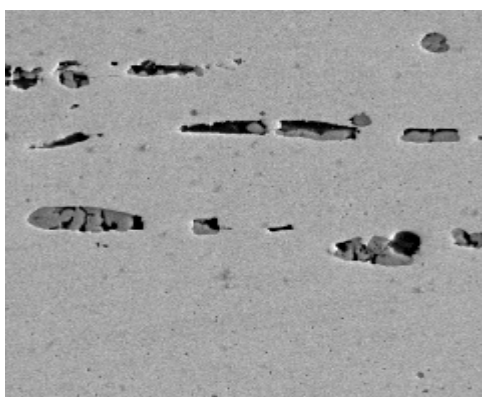
شکل ۲۰: ناخالصی‌های نمونه سرنیزه سه‌پر که منشأ آن سنگ معدن احیا نشده است.
