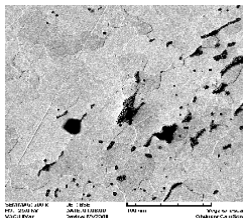
شکل ۱۹: حفرات نمونه سرنیزه سه‌پر که ناشی از خوردگی طی مدت زمان بسیار طولانی است.
