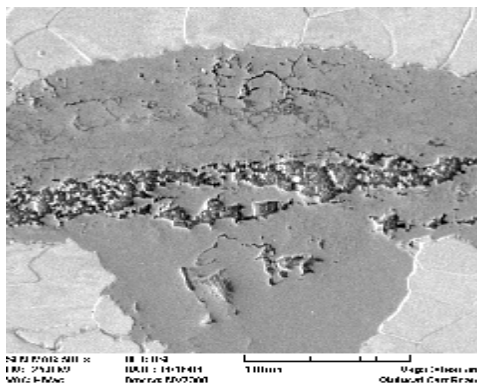
شکل ۲۵: پوشش اکسیدی ترک مرکزی نمونه سرنیزه سه‌پر.
