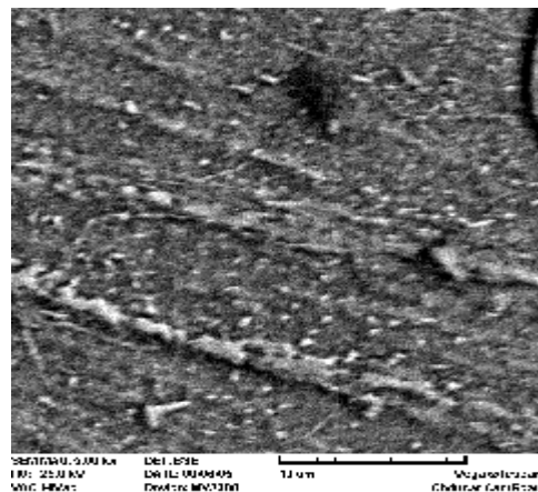
شکل ۱۶: ساختار پرلیتی نمونه میلی‌آهنی.
