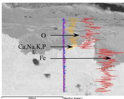
شکل ۲۲: آنالیز خطی پوشش اکسیدی سطح نمونه سرنیزه سه‌پر که مشابه با آنالیز خطی ترک مرکزی نمونه است.
