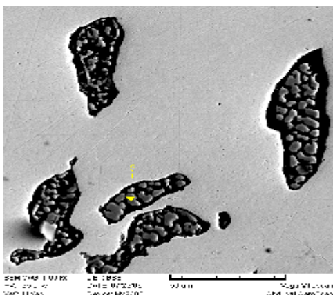
شکل ۲۰: ناخالصی‌های نمونه سرنیزه سه‌پر که منشأ آن سنگ معدن احیا نشده است.
