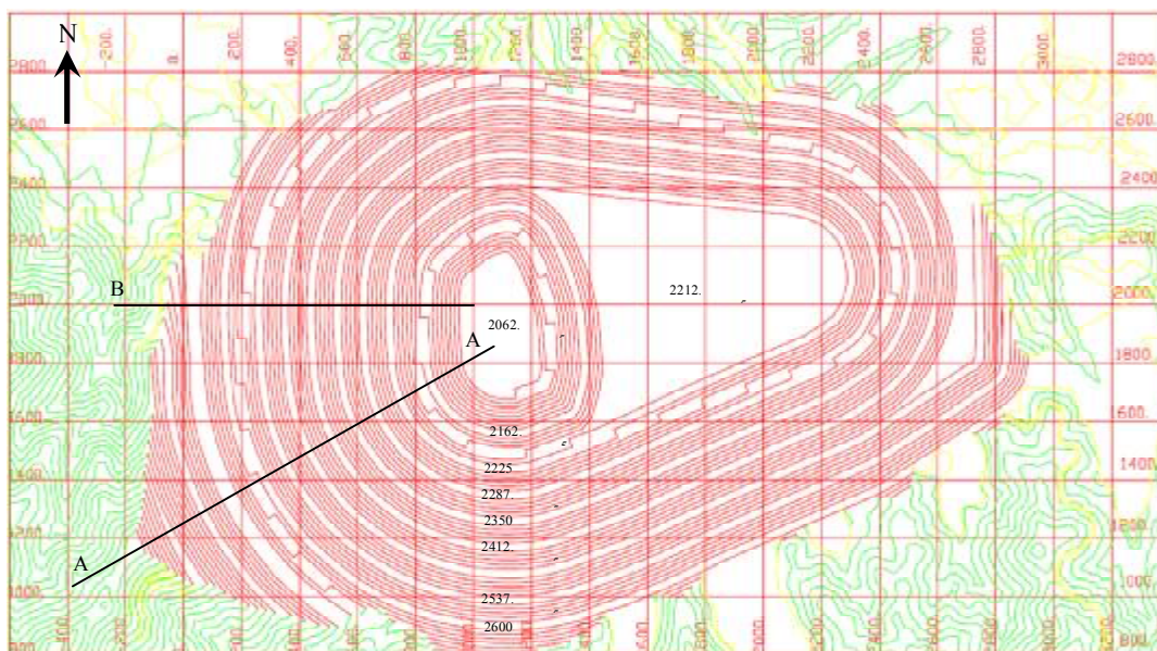
شکل ۳: موقعیت مقاطع انتخابی در کاواک نهایی معدن مس سرچشمه جهت تحلیل.
