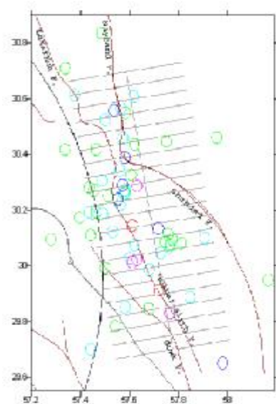
شکل ۳: چشمه‌ی لرزه‌زای ۴.
