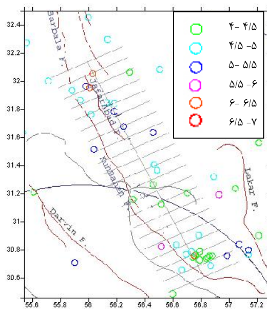
شکل ۲: چشمه‌ی لرزه‌زای ۳.
