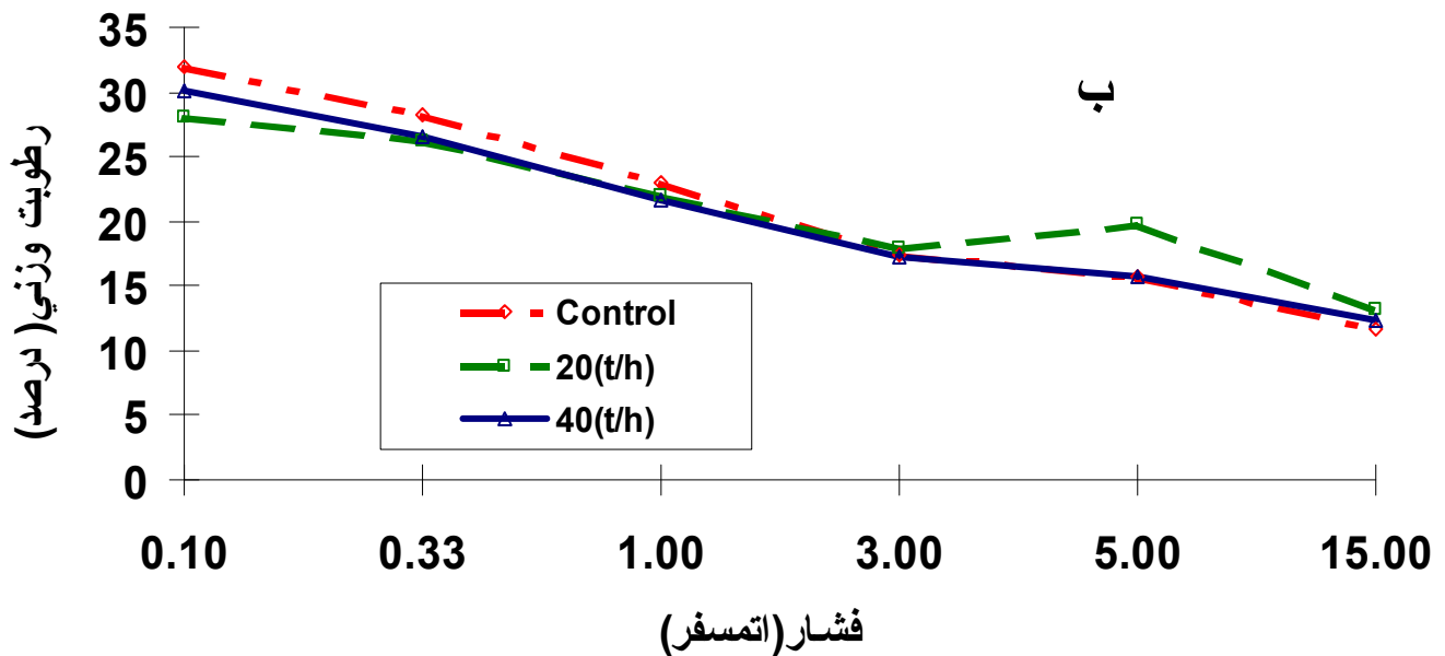
نمودار ۵- منحنی رطوبتی برای تیمارهای مختلف و عمق ۱۵-۰ (الف) و ۳۰-۱۵ (ب)
