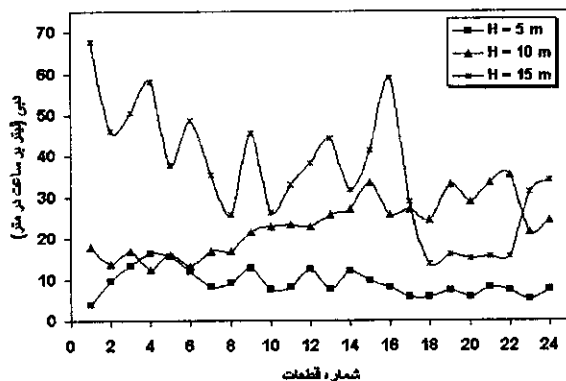
شکل ۱ - تغییرات دبی جریان در طول لوله تراوا در ابتدای آزمایش (۵+ ساعت) در فشارهای مختلف
