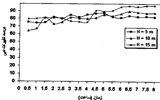
شکل ۱۰ - رابطه تغییرات دبی با زمان در فشارهای مختلف
