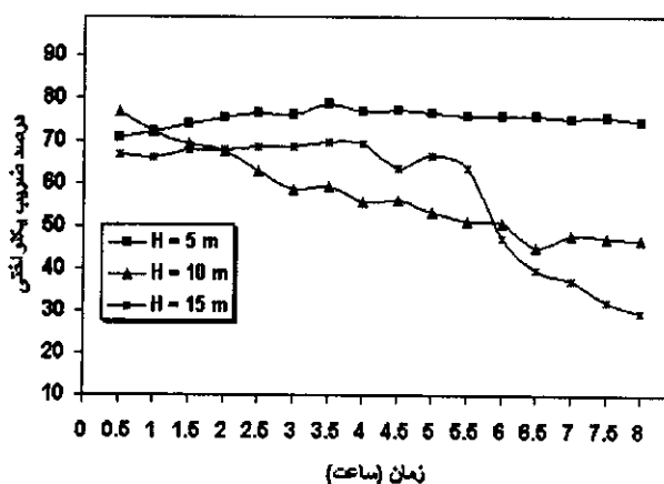
شکل ۹ - تغییرات ضریب یکنواختی با زمان در فشارهای مختلف
