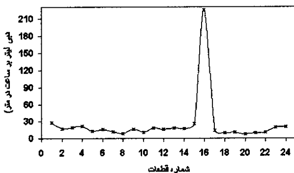
شکل ۳ - تغییرات دبی جریان در طول لوله تراوا در انتهای آزمایش (۸ ساعت) در فشار ۱۵ متر
