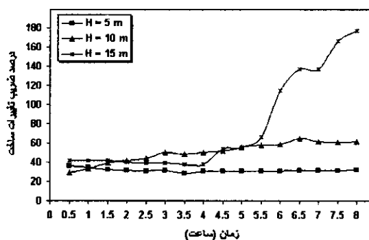
شکل ۷ - تغییرات ضریب تغییرات ساخت با زمان در فشارهای مختلف
