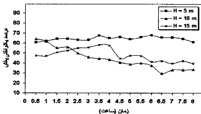
شکل ۸ - تغییرات یکنواختی بخش با زمان در فشارهای مختلف
