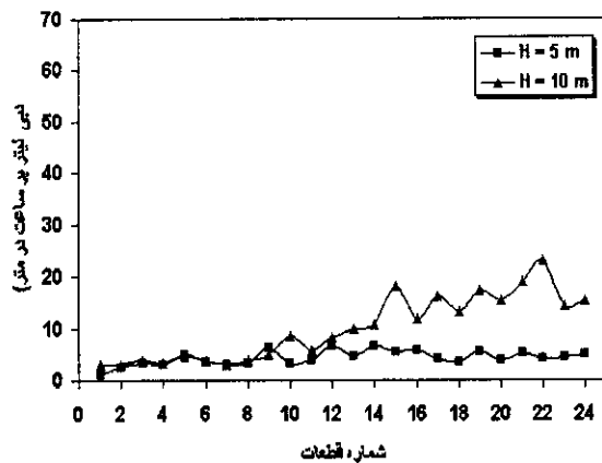
شکل ۲ - تغییرات دبی جریان در طول لوله تراوا در انتهای آزمایش (۸ ساعت) در فشارهای ۵ و ۱۰ متر
