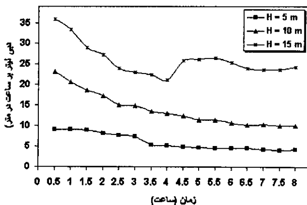
شکل ۴ - تغییرات دبی لوله تراوا با زمان در فشارهای مختلف
