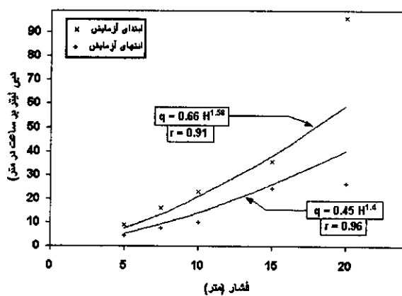
شکل ۵ - معادله توانی رگرسیون بین دبی و فشار در ابتدا و انتهای آزمایش
