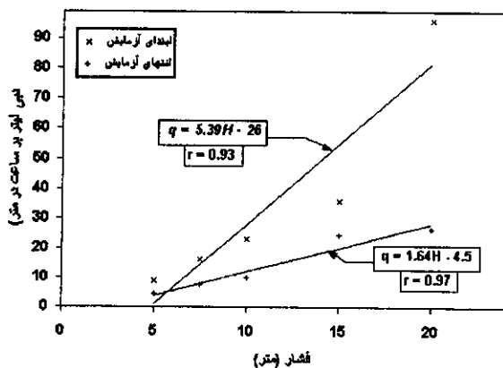
شکل ۶ - معادله خطی رگرسیون بین دبی و فشار در ابتدا و انتهای آزمایش
