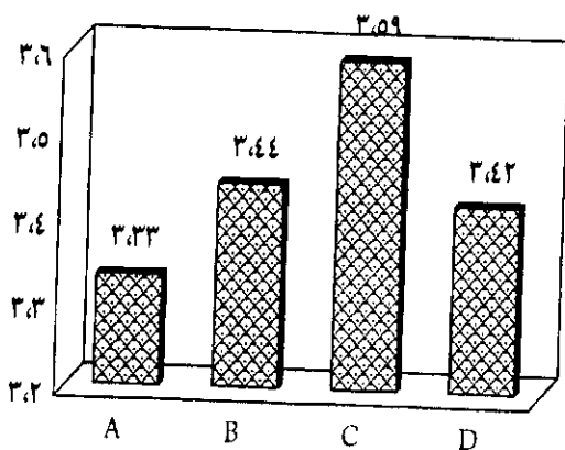
نمودار ۱: فراوانی نسبی اقدام به خودکشی بر اساس چهار دوره ماه قمری در طی سه سال
