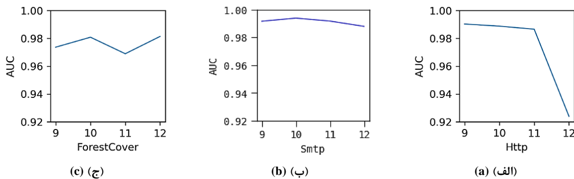
(شکل ۷): مقدار AUC حاصل شده به‌وسیله روش پیشنهادی با استفاده از اندازه‌های مختلف پنجره در مقیاس لگاریتمی (محور افقی) بر روی سه مجموعه داده HTTP، SMTP و Covertypes (Figure-7): AUC values obtained by the proposed method using different window sizes in logarithmic scale (horizontal axis) on three datasets (a) HTTP, (b) SMTP and (c) Covertypes
