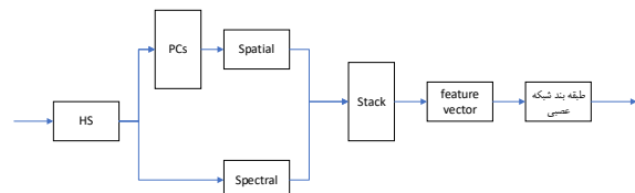
(شکل ۴): استفاده از طبقه‌بند شبکه عصبی در روش زیر هم
