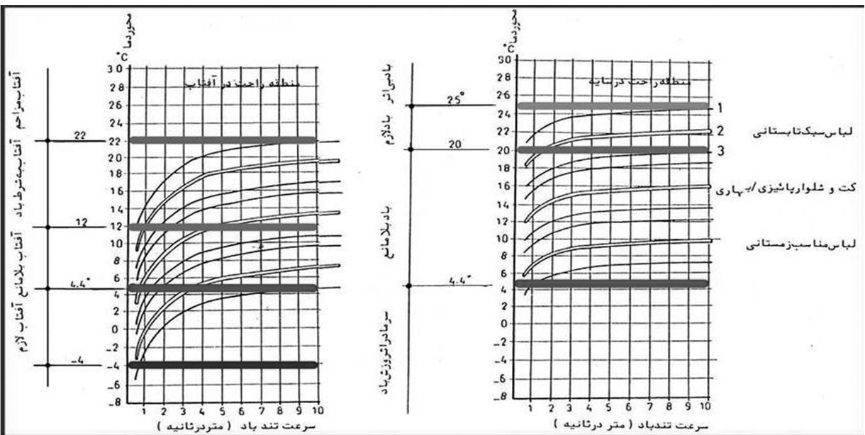
تصویر ۲: معیار آسایش پدین واردن برای فضاهای باز. مأخذ: (طاهیان، ۱۳۶۹)
