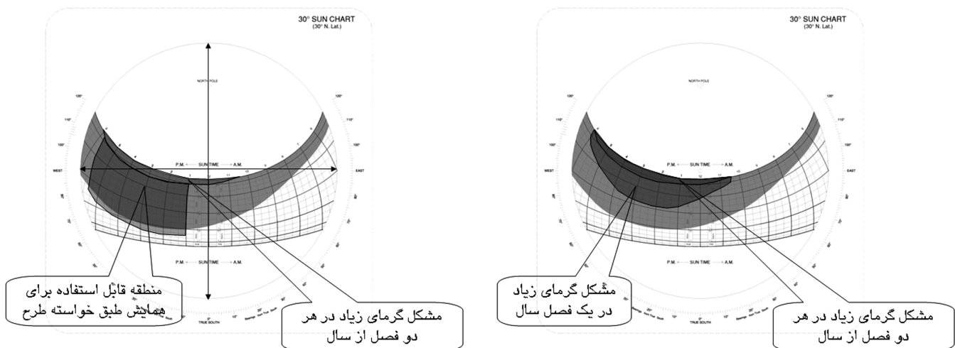
تصویر ۵- راست: نقشه مسیر خورشید بم با موقعیتهای مختلف نیاز به سایه روی آن چپ: مواقع منتخب نیاز به سایه روی نقشه مسیر خورشید بم مأخذ: (نگارنده)
