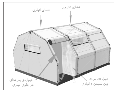
تصویر ۱۹ - وضعیت قرارگیری در و پنجره ها و دیواره های جداکننده.
