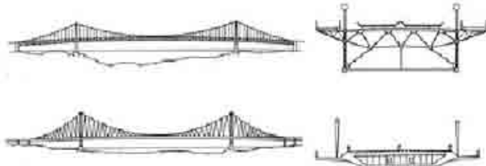
تصویر ۱۰- تغییر در طراحی پل معلق، مقایسه طرح و مقطع عرضی بین پل فورث رود ۱۱ (۱۹۶۴) و پل سون ۱۲ (۱۹۶۶). ماخذ: (Art of Structural Design, Holgate, A. 1986)
