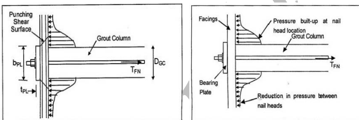
تصویر ۱۹- الف- توزیع فشار تیپ در پوسته بتنی. ب- برش تیپ در صفحه اتصال باربر. مأخذ: (Shaw - Shong, 2005)
