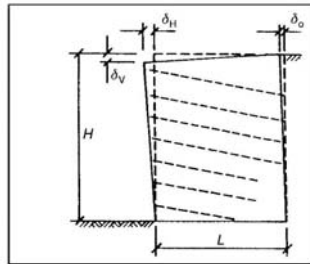
تصویر ۲۴ - تعاریف تغییر مکان‌های \delta_o ، \delta_v ، \delta_h مأخذ: (PULLER, 2003, 88)
