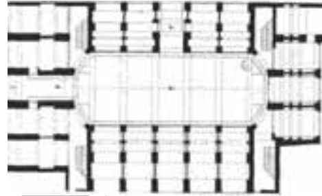
نقشه ۵- پلان تیمچه اکبریان. (مأخذ: نگارندگان)
