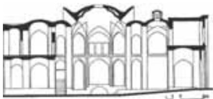
نقشه ۱۰-ب: مقطع تیمچه گمرک. (مأخذ: نگارندگان)
