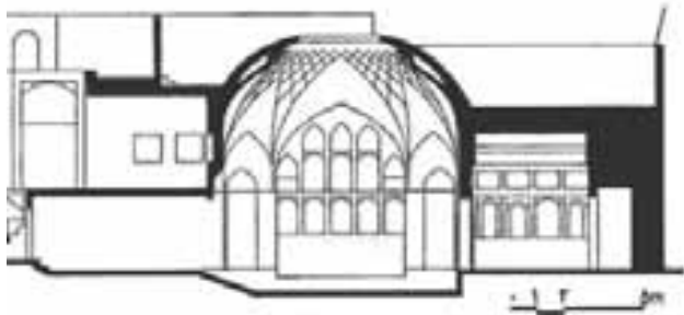
نقشه ۹- ب: مقطع تیمچه علی آقا. (مأخذ: نگارندگان)
