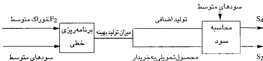
نمودار ۳ دیاگرام بلوکی محاسبه S_2 و S_4
