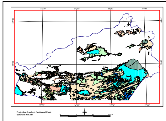
شکل ۲۳ الف- مجموع مناطق مساعد برای کشاورزی و زیستی؛ ب- مجموع پلایاها در استان سمنان که بدون شرایط زیستی است
