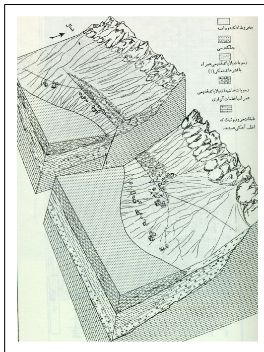
شکل ۲ بلوک دیاگرام نشانگر روابط میان زمین‌شناسی و لندفرمهای حاشیه شمالی پلایای دامغان است [۱].
