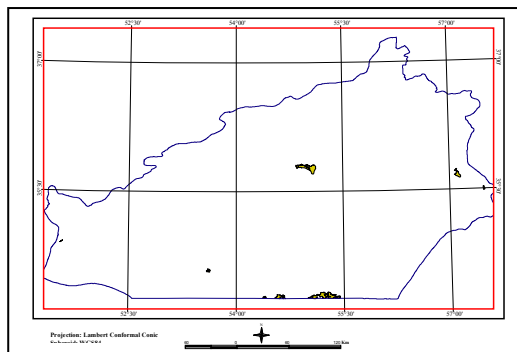
شکل ۱۸ الف- وجود تپه ماسه‌ها در مرز جنوبی و در مرز شرقی به همراه رسوبات نمکی؛ ب- پراکندگی سنگفرش بیابانی در استان سمنان.
