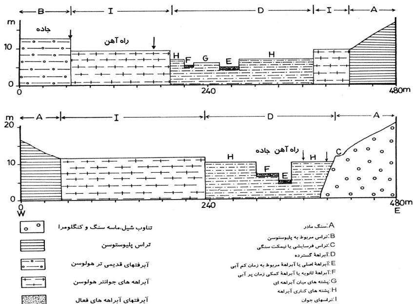
شکل ۶ مقاطع ژئومورفولوژیکی رودخانه پیام چای
