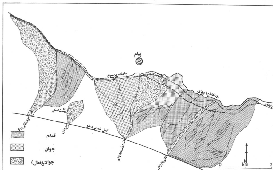
شکل ۸ نقشه مخروط افکنه‌های بخش مرتفع گردنه پیام و بخشهای مختلف آنها
