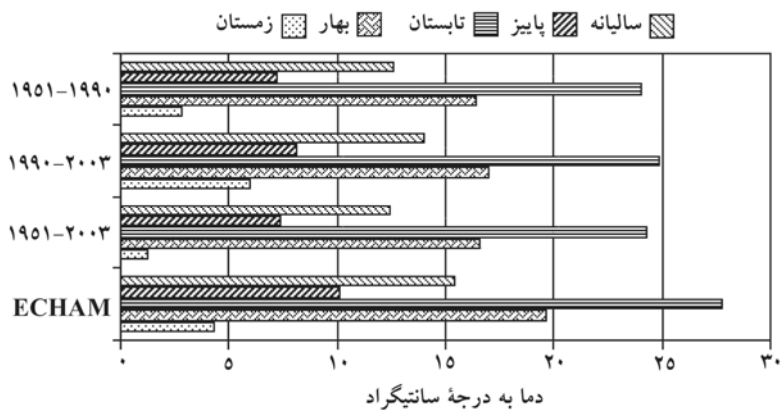
شکل ۹ نمودار تغییرات دمای فصلی و سالیانه فعلی نسبت به شبیه‌سازی مدل ECHAM در وضعیت دوبرابر شدن CO 2 جو
