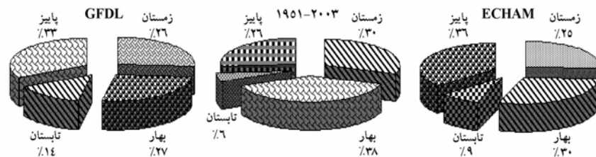
شکل ۱۲ توزیع فصلی و تغییر رژیم بارش شبیه‌سازی شده از مدلها نسبت به دوره ۱۹۵۱-۲۰۰۳ ایستگاه تبریز
