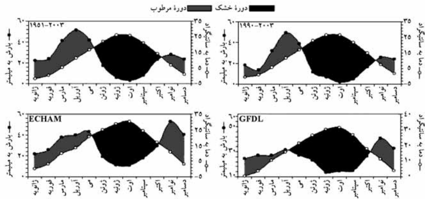
شکل ۱۴ مدل‌های آمبروترمیک فعلی و شبیه‌سازی شده تبری از طریق مدل‌های گردش جهانی GFDL و ECHAM۴
