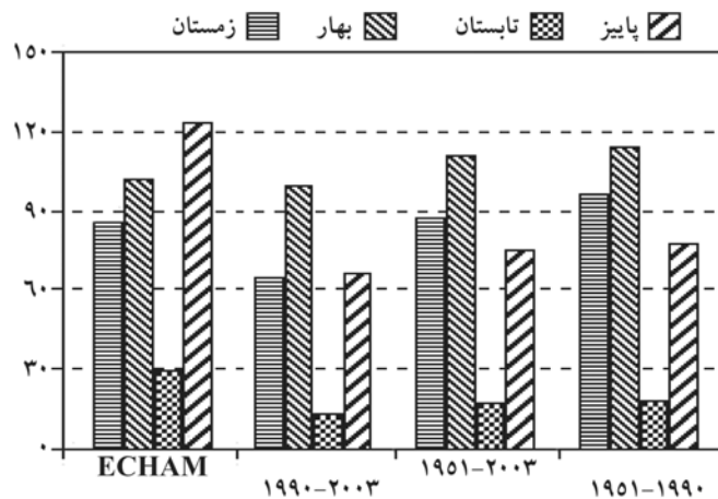
شکل ۱۰ تفاوت‌های فصلی بارش فعلی با بارش شبیه‌سازی شده از مدل ECHAM
