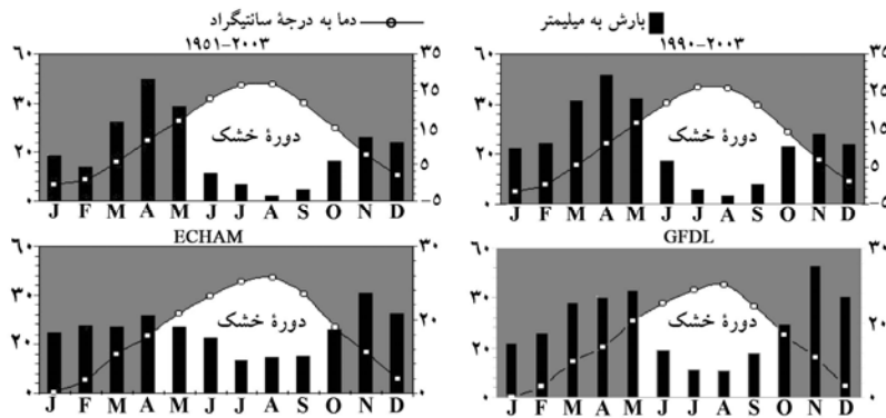
شکل ۱۵ مدل‌های اقلیم‌نگاشت (کلیماگرام) فعلی و شبیه‌سازی شده تبری در وضعیت دوبرابر شدن دی‌اکسیدکربن جو
