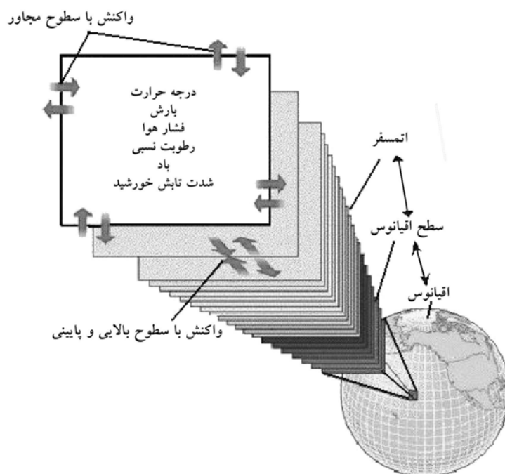
شکل ۱ نمایش شماتیک و ساده شده‌ای از یک مدل گردش جهانی پیوندی جوی- اقیانوسی [۲، ص ۲۵۳]
