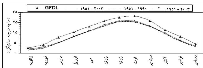
شکل ۳ مدل خطی تغییرات ماهیانه درجه حرارت فعلی و شبیه‌سازی شده از مدل GFDL
