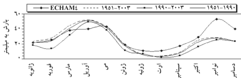
شکل ۸ مدل خطی تغییرات ماهیانه بارش فعلی در مقاطع ماهیانه، فصلی، سالیانه و شبیه‌سازی شده از مدل ECHAM
