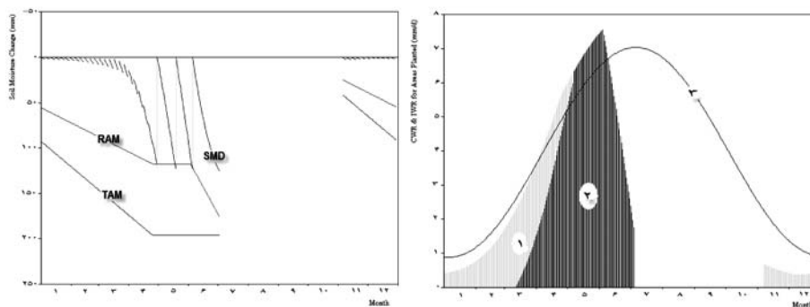
شکل ۸ نمودار نیاز آبی محصول و کمبود رطوبت خاک در ایستگاه سرپیل زهاب
