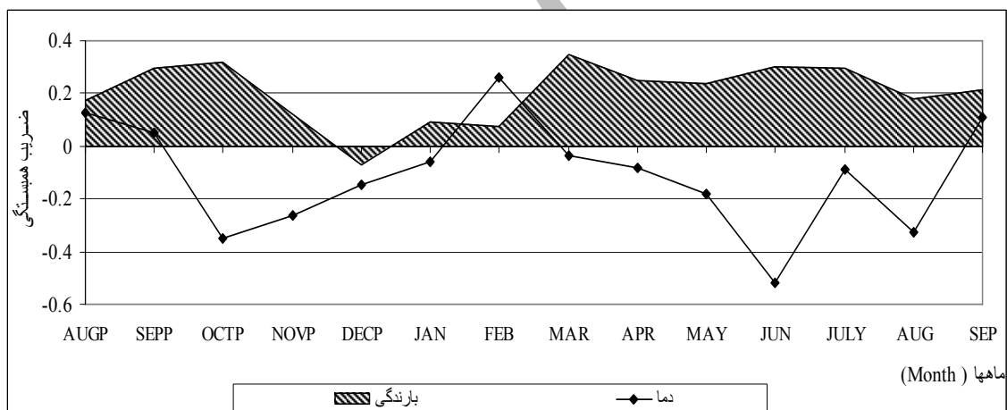
شکل ۹- همبستگی بین پهنی دوایر رویشی درختان کاج پارک چیتگر با دما و بارندگی ایستگاه چیتگر
